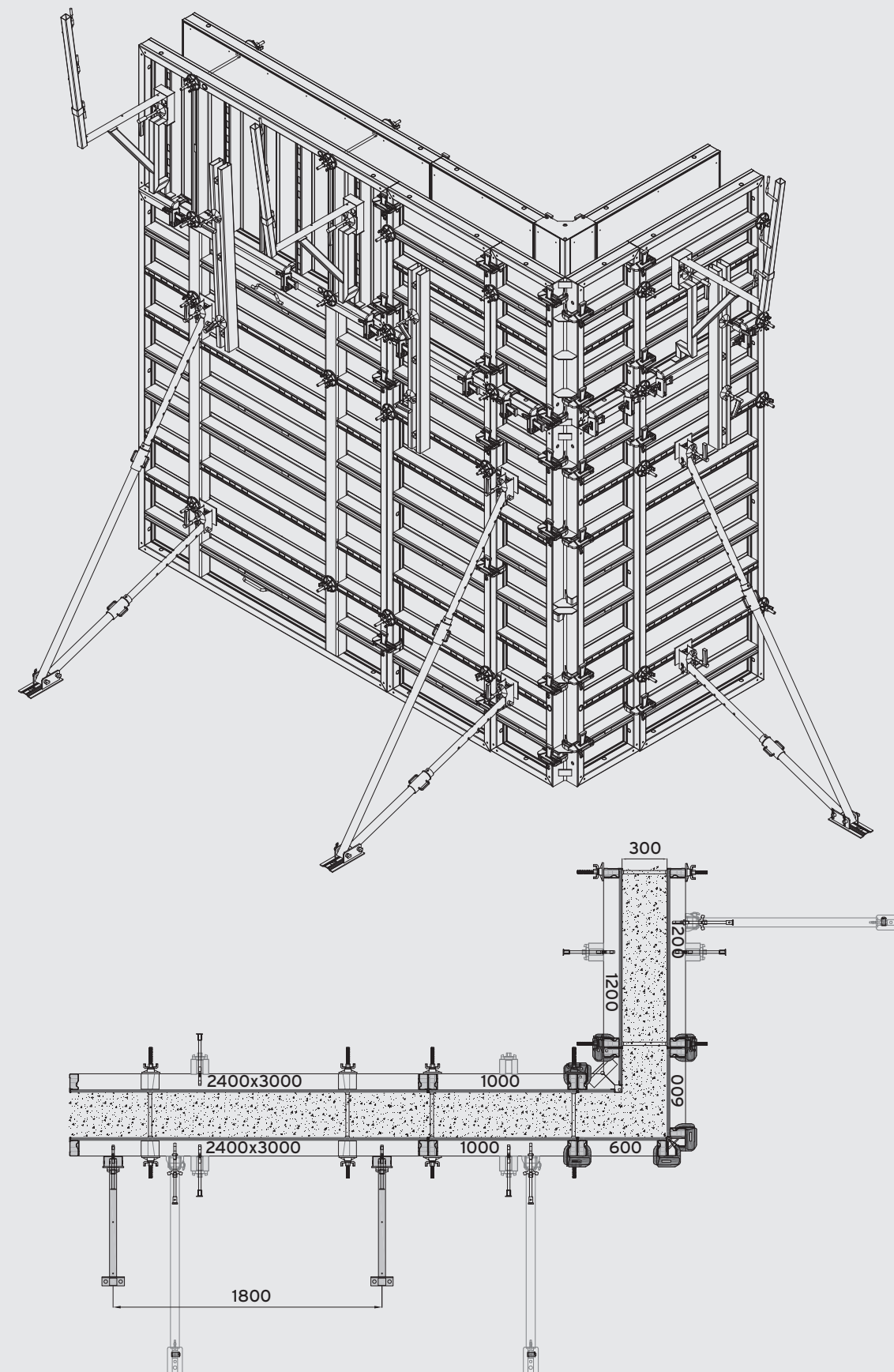
90° ANGLE WITHOUT COMPENSATION (USING ANGULAR FORMWORK ELEMENTS) ANGOLI A 90° SENZA COMPENSAZIONE (USANDO ELEMENTI ANGOLARI)
